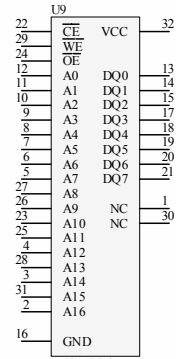
RAM28F101 Pamięć o organizacji 128kBx8
