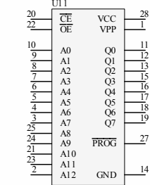
ROM27C64 Pamięć o organizacji 8kBx8
