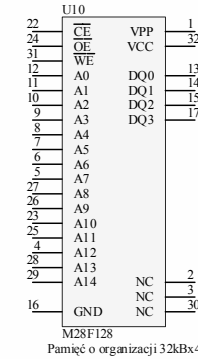
M28F128 Pamięć o organizacji 32kBx4
