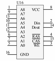
41256 Pamięć o organizacji 256kBx1
