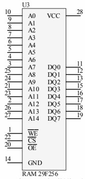
RAM 29F256 Pamięć o organizacji 32kBx8
