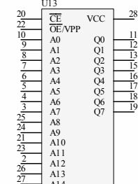
ROM27C512 Pamięć o organizacji 64kBx8
