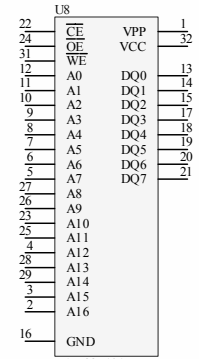
RAM28F101 Pamięć o organizacji 128kBx8
