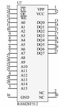
RAM28F512 Pamięć o organizacji 64kBx8
