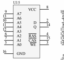
4164 Pamięć o organizacji 64kBx1
