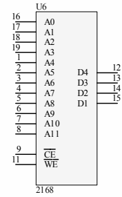
Pamięć o organizacji 4kBx4
