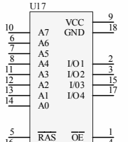
71C464 Pamięć o organizacji 64kBx4
