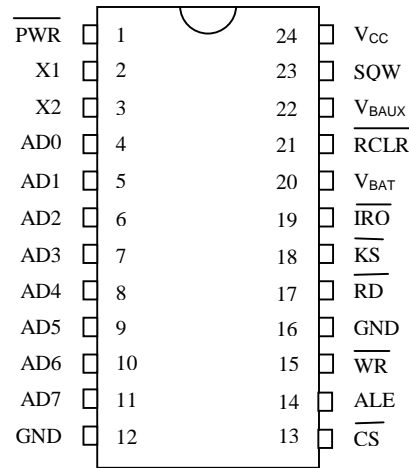
DS1685 24-Pin DIP DS1685S 24-Pin SOIC DS1685 24-Pin TSSOP
