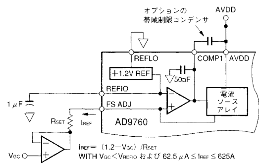
図44．両電源ゲイン制御回路
