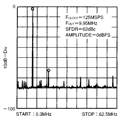
図36 . 1波のSFDR
