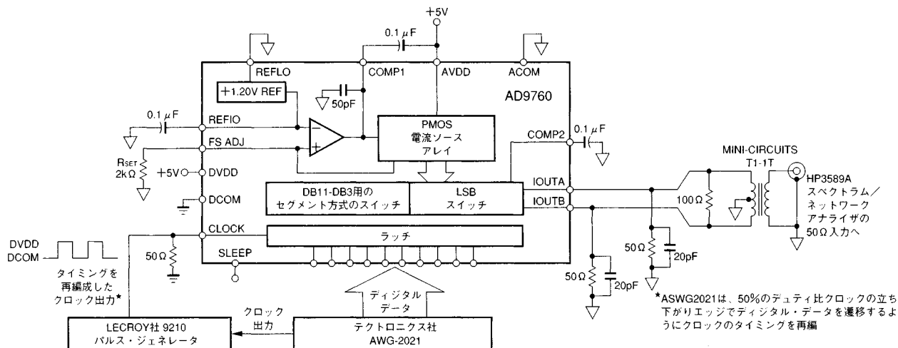
図2. 基本AC特性テスト用の構成
