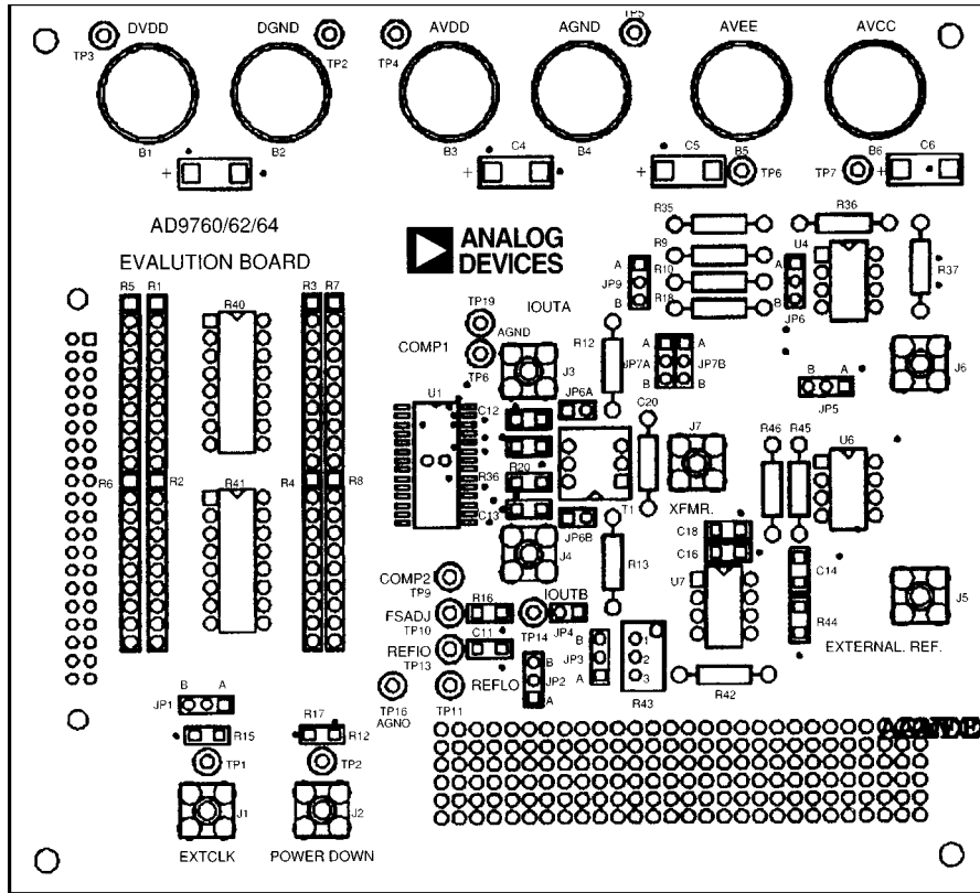
図60. シルクスクリーン層 - 上
