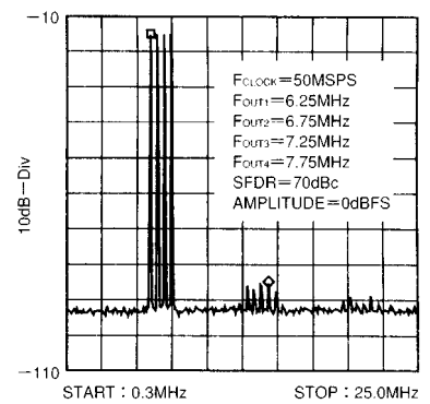
図20. 4波のSFDR
