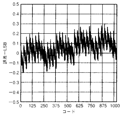
図15. 代表的なINL
