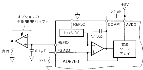
図40．内部リファレンス構成
