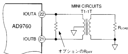
図50．トランスを使用した差動出力
