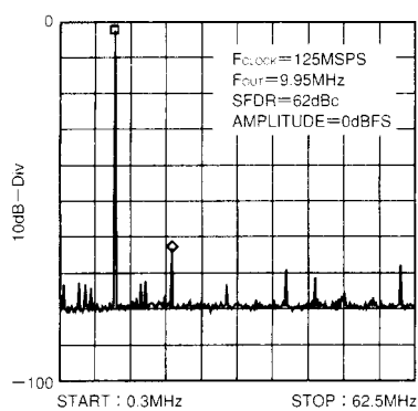
図18. 1波のSFDR
