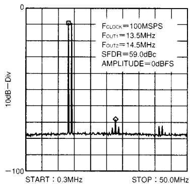
図37 . 2波のSFDR
