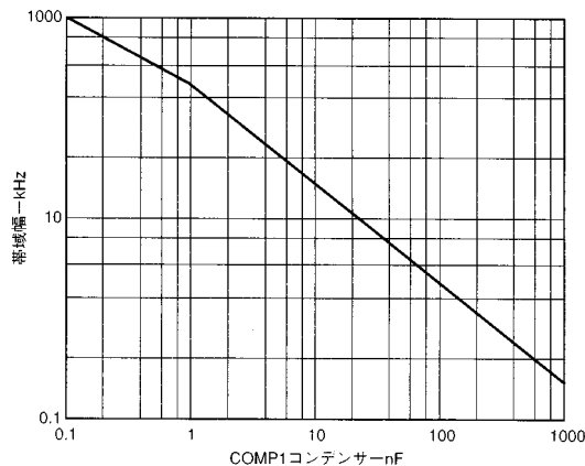
図42．外部COMP1コンデンサと - 3dB帯域幅
