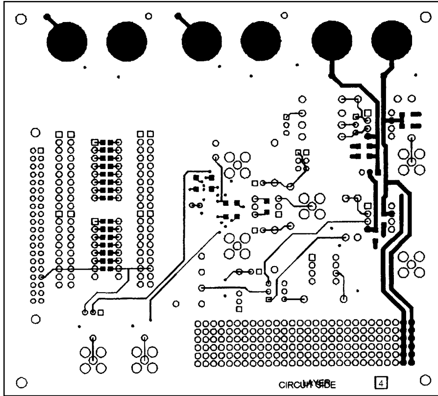
図64 . プリント回路基板のハンダ面(第4層)
