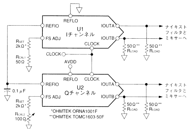
図57 . 2個のAD9760を使用したベースバンドQAM構成
