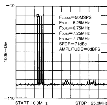
図38 . 4波のSFDR
