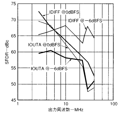
図14. 差動方式とシングル・エンド方式の SFDRと f_{\text{OUT}}
