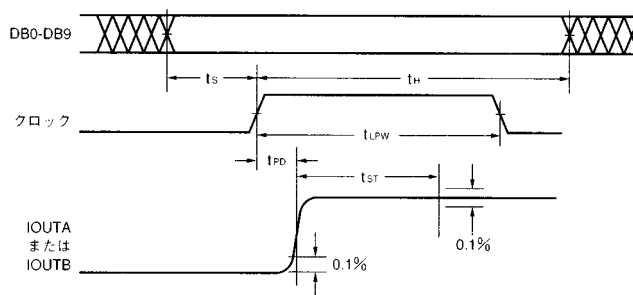
図1. タイミング図
