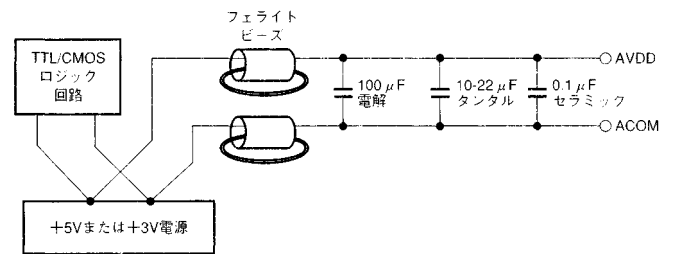
図55 . +5 Vまたは+3 V単電源アプリケーション用の差動LCフィルタ
