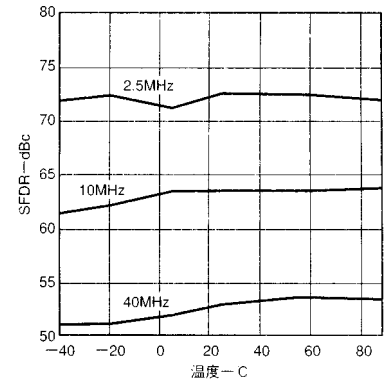
図17. SFDRと温度 @ 100MSPS、0dBFS
