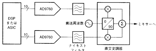
図56 . 代表的なQAM構成
