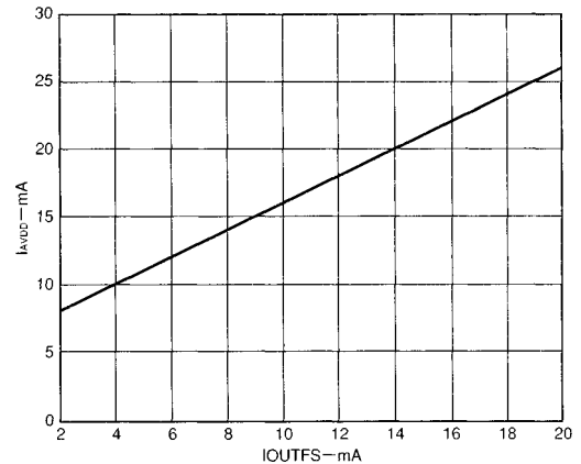
図47. I_{AVDD} と I_{OUTFS}
