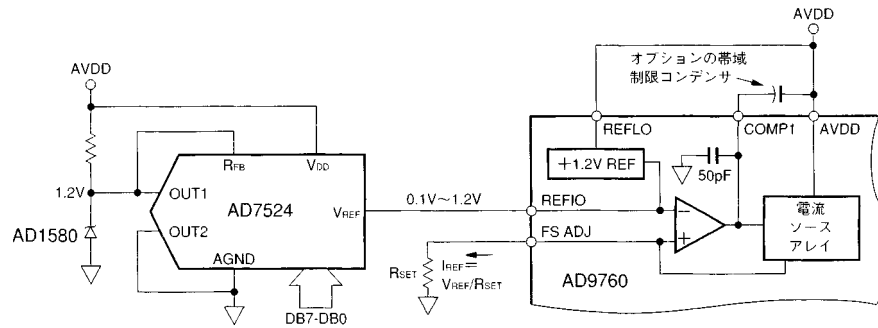
図43．単電源ゲイン制御回路
