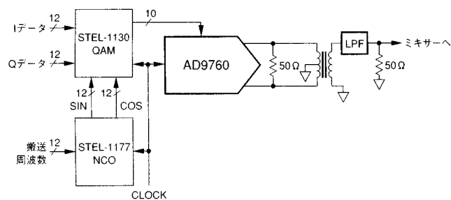
図58 . デジタルQAM構成
