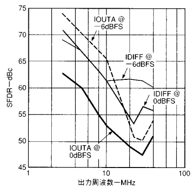
図32 . 差動方式とシングル・エンド方式の SFDRと f_{\text{OUT}}
