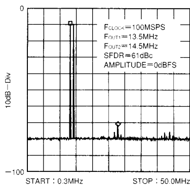
図19. 2波のSFDR
